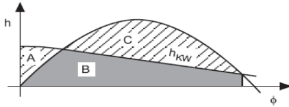
h_{KW} = Kurve der krängenden Hebelarme infolge seitlichen Winddrucks
